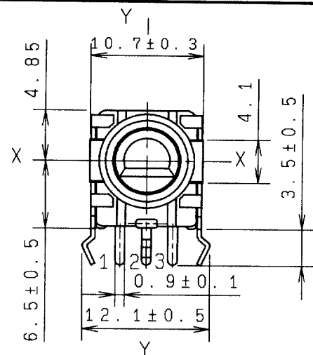
軸はセンター位置を示す SHAFT SHOWN IN CENTER POSITION
